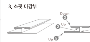
3. 소빗 마감부
