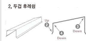
2. 두겹 후레싱
