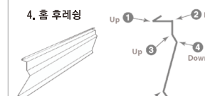
4. 홈 후레싱
